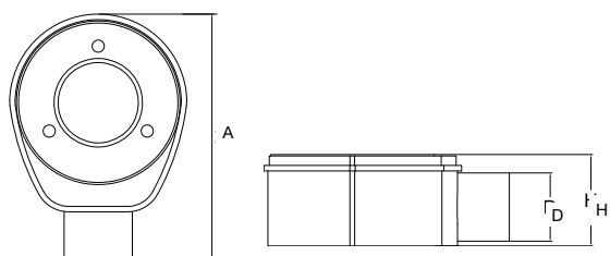
CORPO SIFONATO
